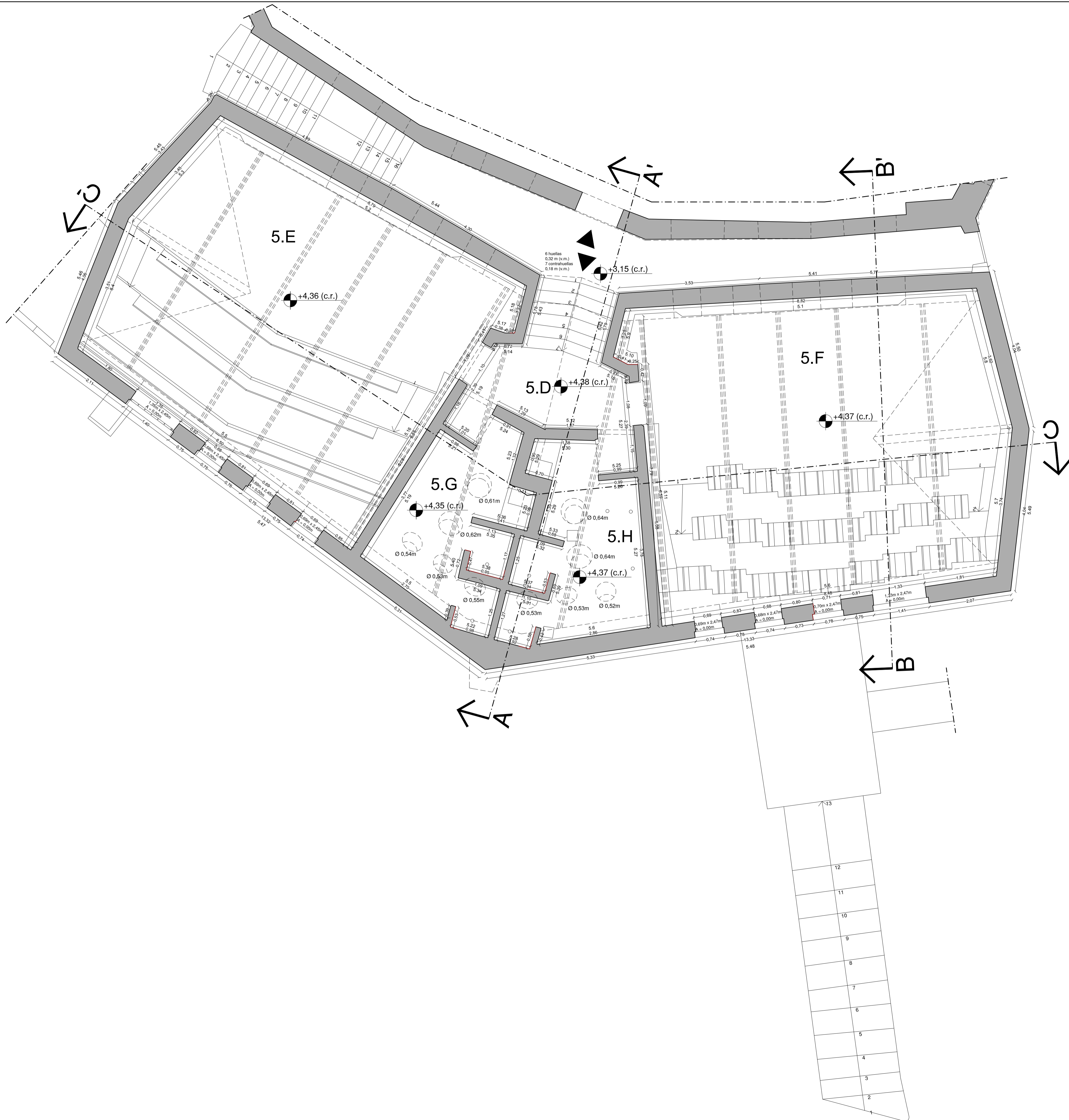
Planta a cota +5,30 (c.r.)
