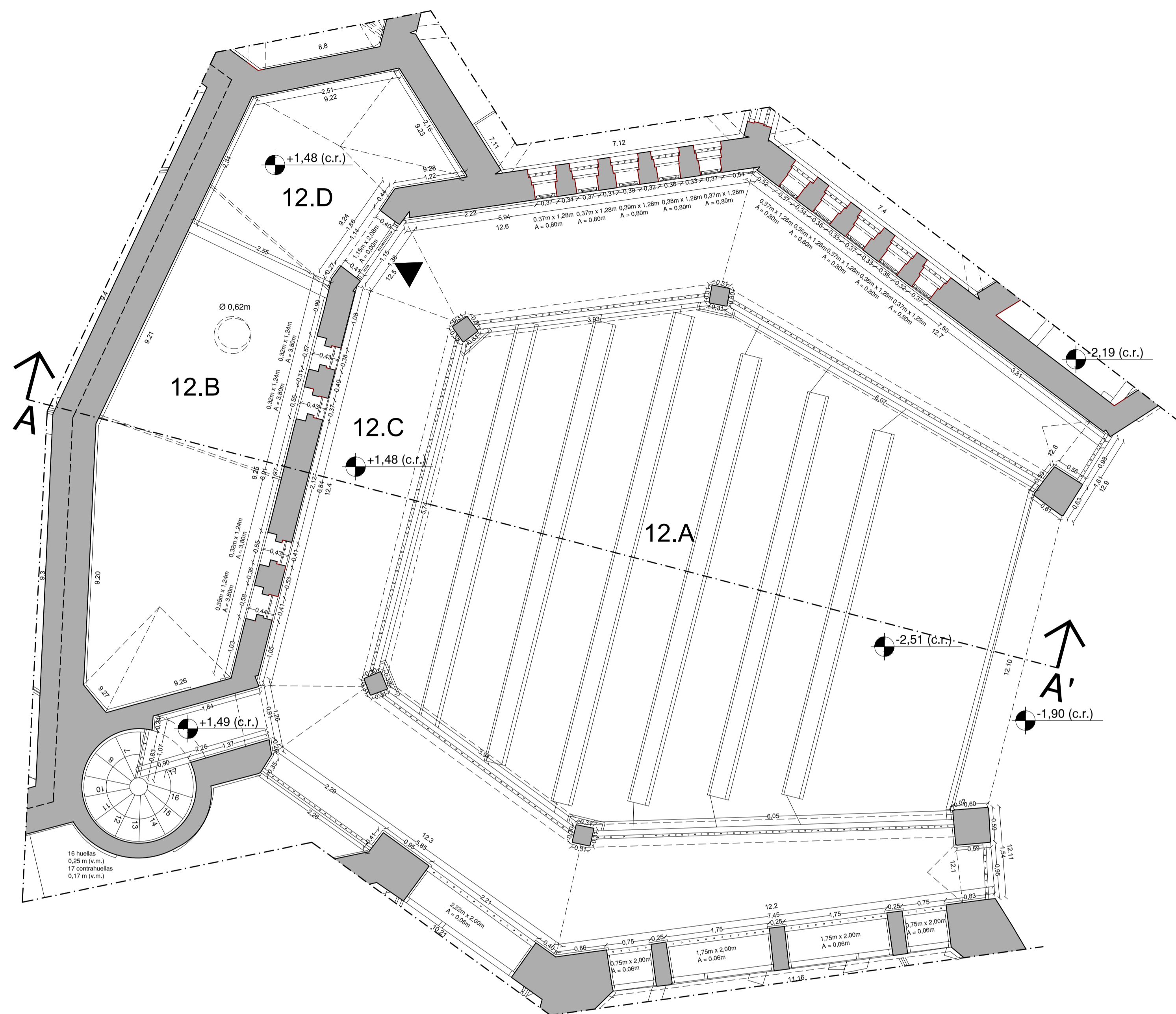
Planta a cota +3,50 (c.r.)
