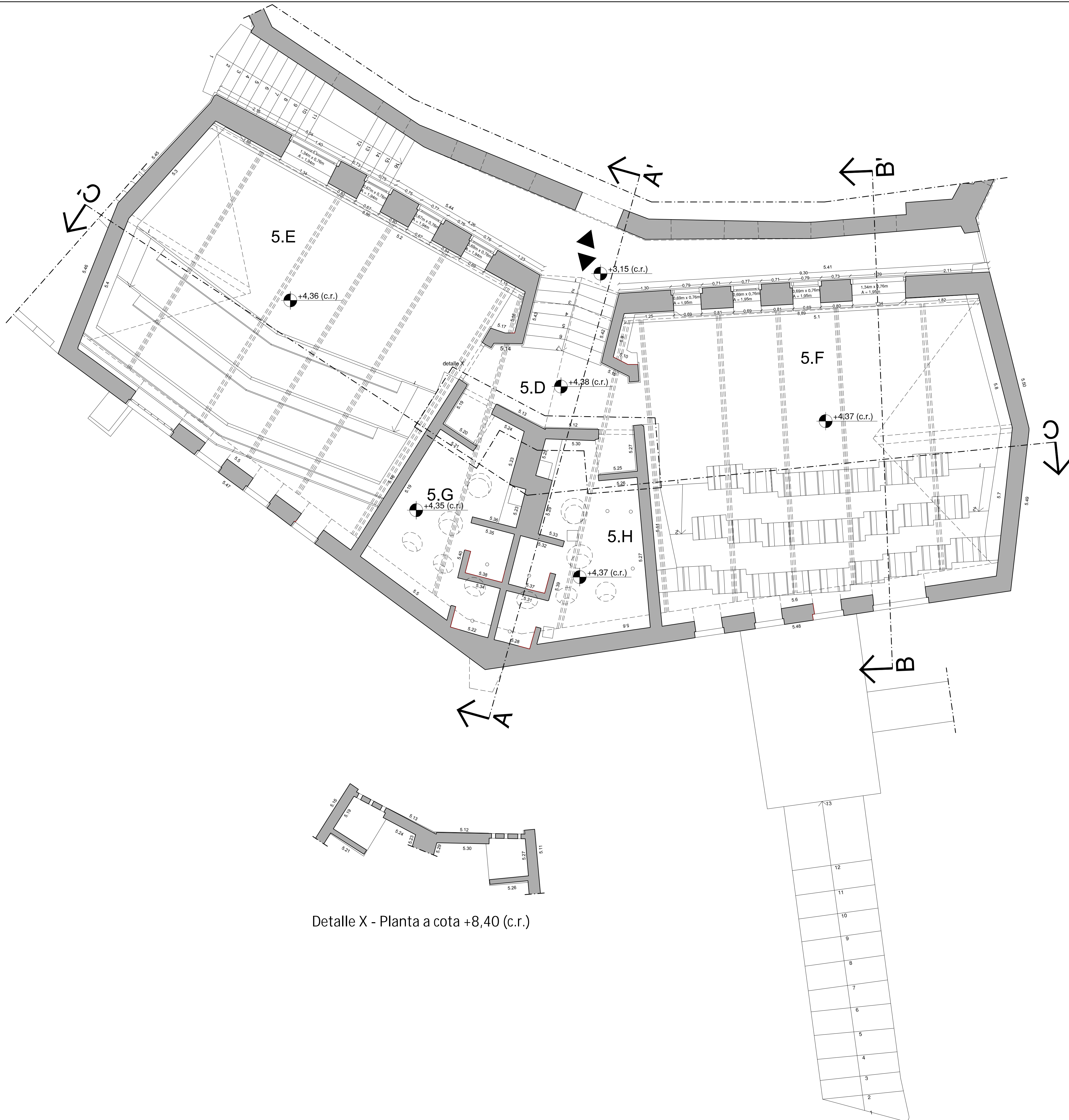
Planta a cota +6,70 (c.r.)
